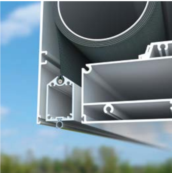
La barre de charge disparaît dans le caisson
