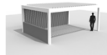
Paroi fixe Linius : sur toute la hauteur de passage ou à une hauteur spécifique + paroi fixe Linarte
